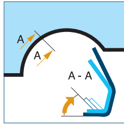
Radhausflansch, zweilagig 双层轮罩法兰
