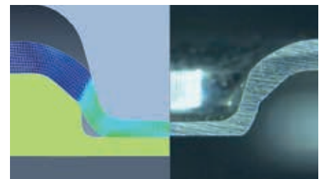
Ideale Werkzeuggeometrien durch Simulation / 通过仿真实现理想的模具几何结构
