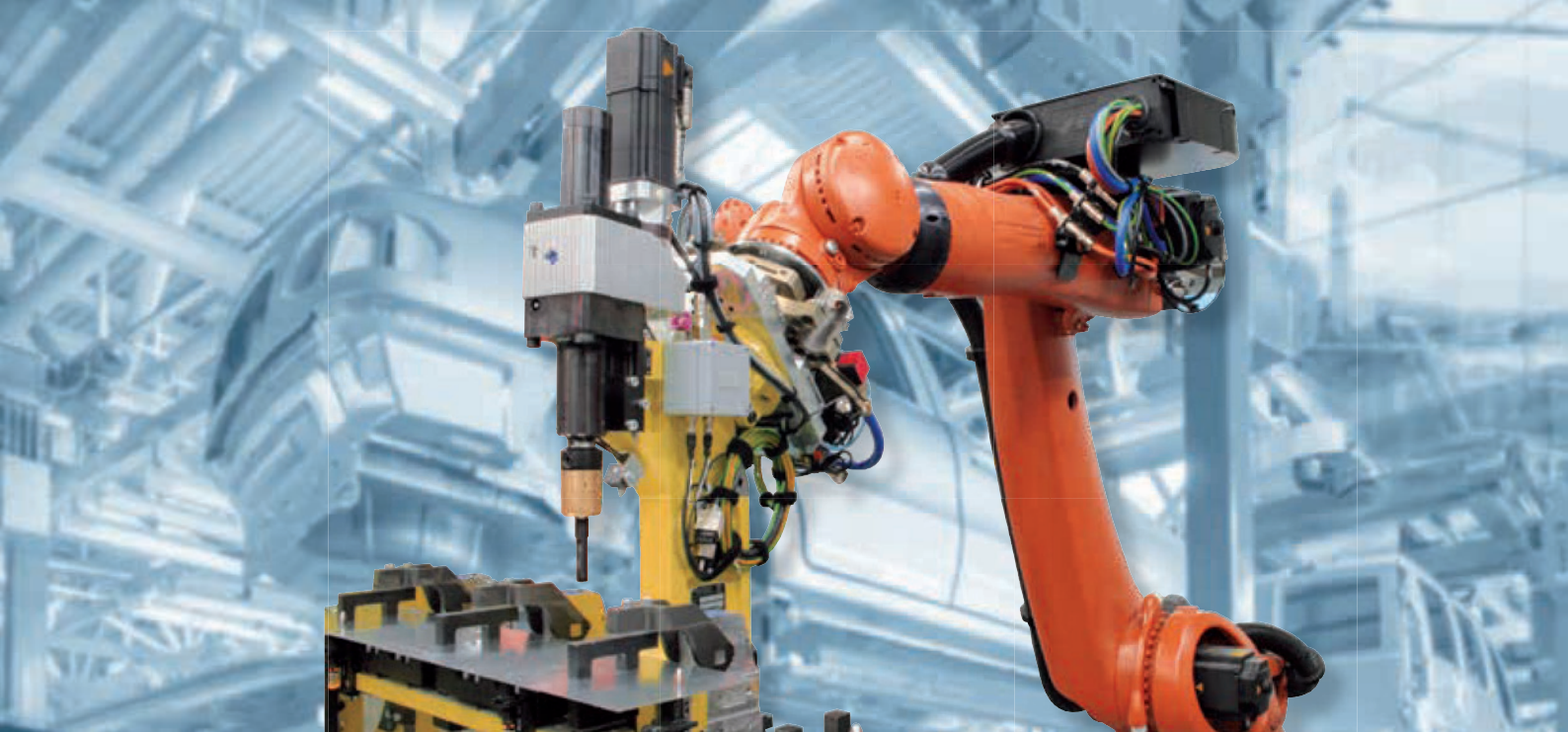
Servomotorisches Clinchsystem mit Prozessüberwachung und Visualisierung / 伺服电动咬合连接系统
