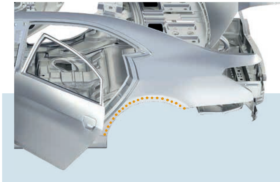
Radhausflansch, zweilagig 双层轮罩法兰
