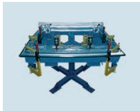
Beispiel einer Falzvorrichtung, kundenseitig beizustellen. 客户提供的折叠装置示例
