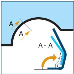
Radhausflansch, einlagig 单层轮罩法兰
